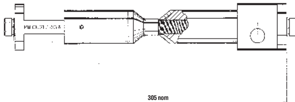
Socket OLI
