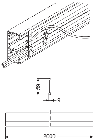
Divider
