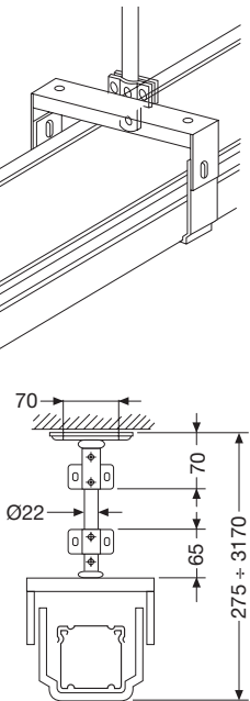
Conduit Ø 22 mm
