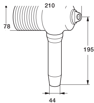
Elbow KAP 300 U.
