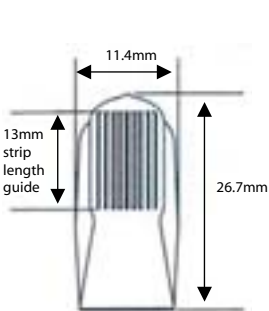
Scotchlok™ Y Connector
