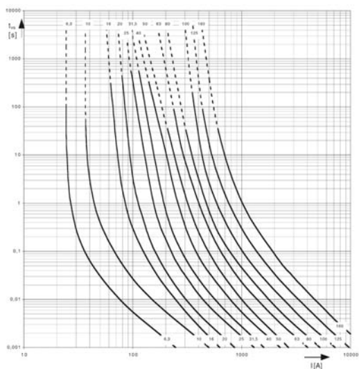
Fig.4 3/7,2 kV
