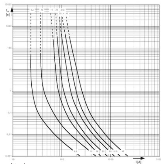
Fig.6 10/24 kV 6,3 A-40 A
